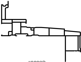
#9698B Cadre 4 1/2" avec moulure à brique intégrée 4 1/2" PVC frame, built-in brick moulding
