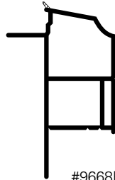
#9668E Moulure à brique en PVC 2", fermée 2" closed PVC brick moulding
