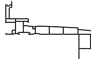
#9800MD Cadre en PVC avec moulure à brique intégrée 5 5/8" (Structurale seulement) 5 5/8" PVC frame, built-in brick moulding (Structural only)
