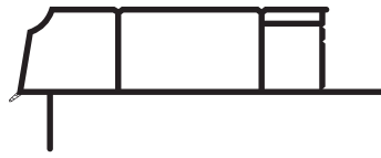
#9468 Moulure à brique 4" en PVC 4" PVC brick moulding
