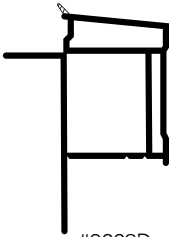
#9668D Moulure à brique en PVC 1 1/2", fermée 1 1/2" closed PVC brick moulding
